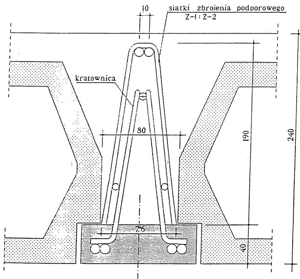
przekrój poprzeczny przez zebro w strefie podporowej
