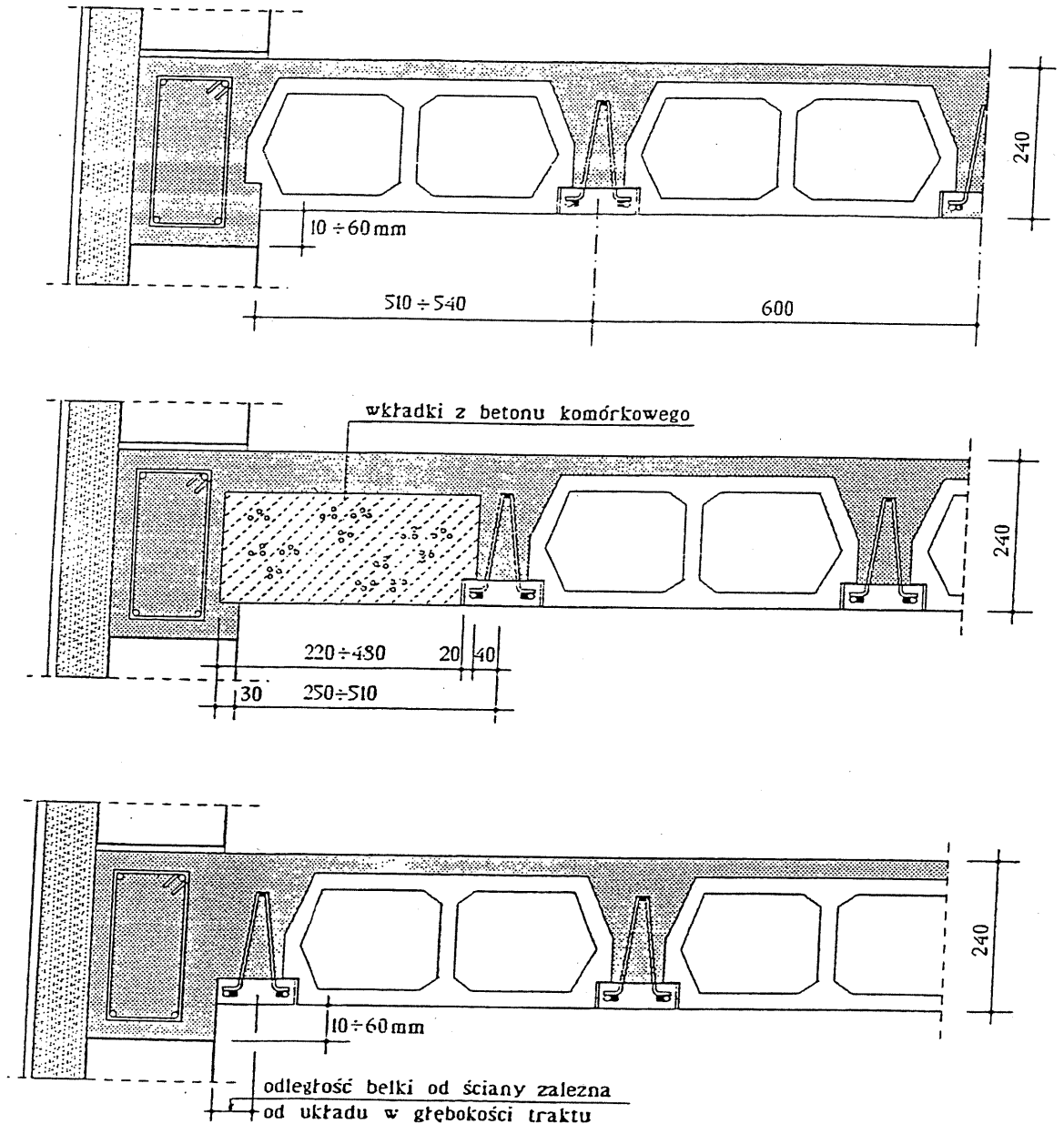
Z6-2. Sposób układania pustaków przy ścianach równoległych do belek
